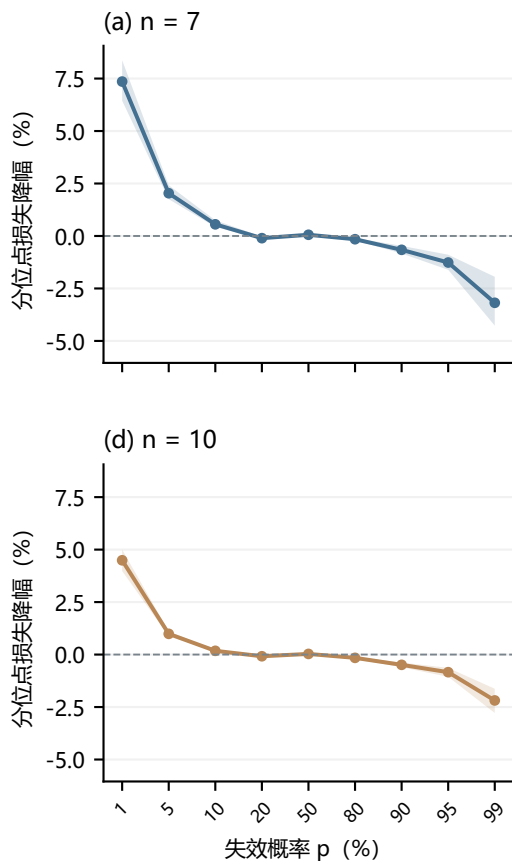
铝合金疲劳寿命 (101个)
