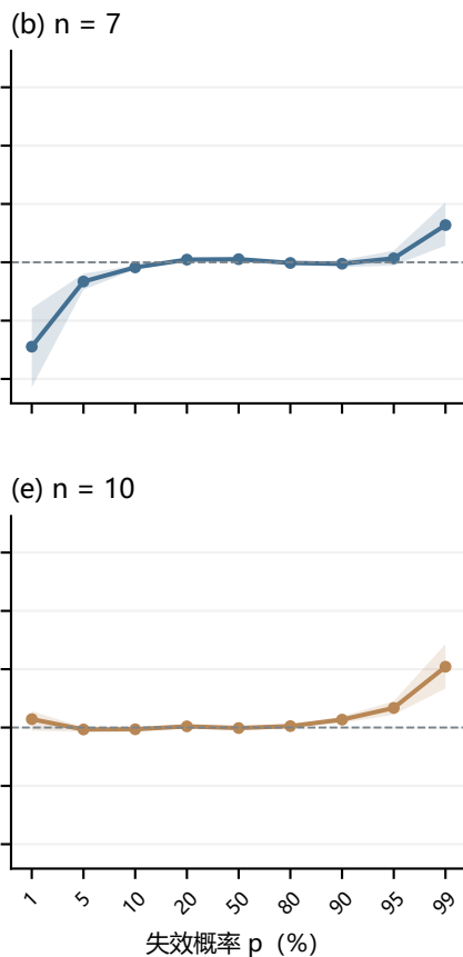
转子寿命 (20个)
